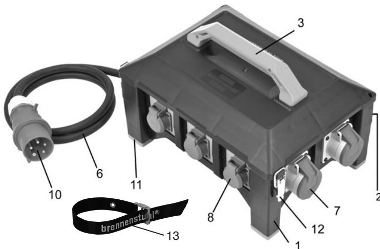
Afb. A, voorbeeld stroomverdeler BSV 5 3/6 N560
