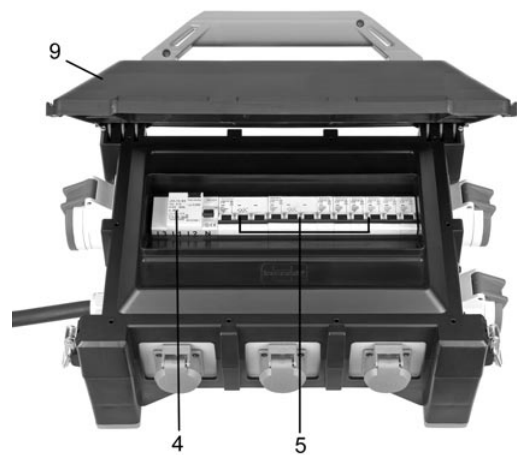
Afb. B, voorbeeld stroomverdeler BSV 5 3/6 N560
