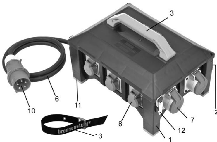
Abb. A, Bsp. Stromverteiler BSV 5 3/6 N560
