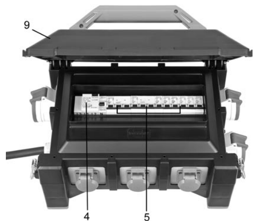
Afb. B, voorbeeld stroomverdeler BSV 5 3/6 N560
